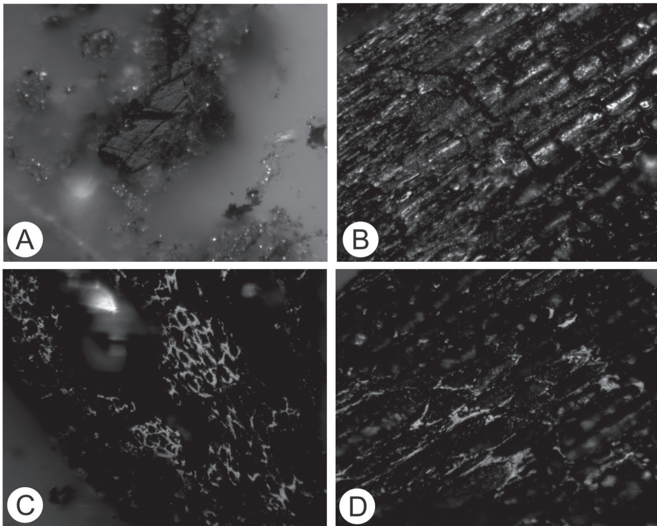
Figura 3. Fusenita. A , amostra inserida em resina, 100 x; B , tecido epidérmico carbonizado, 300 x; C-D , células impregnadas de fusenita, 500 x.
